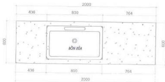
MẶT BẰNG
