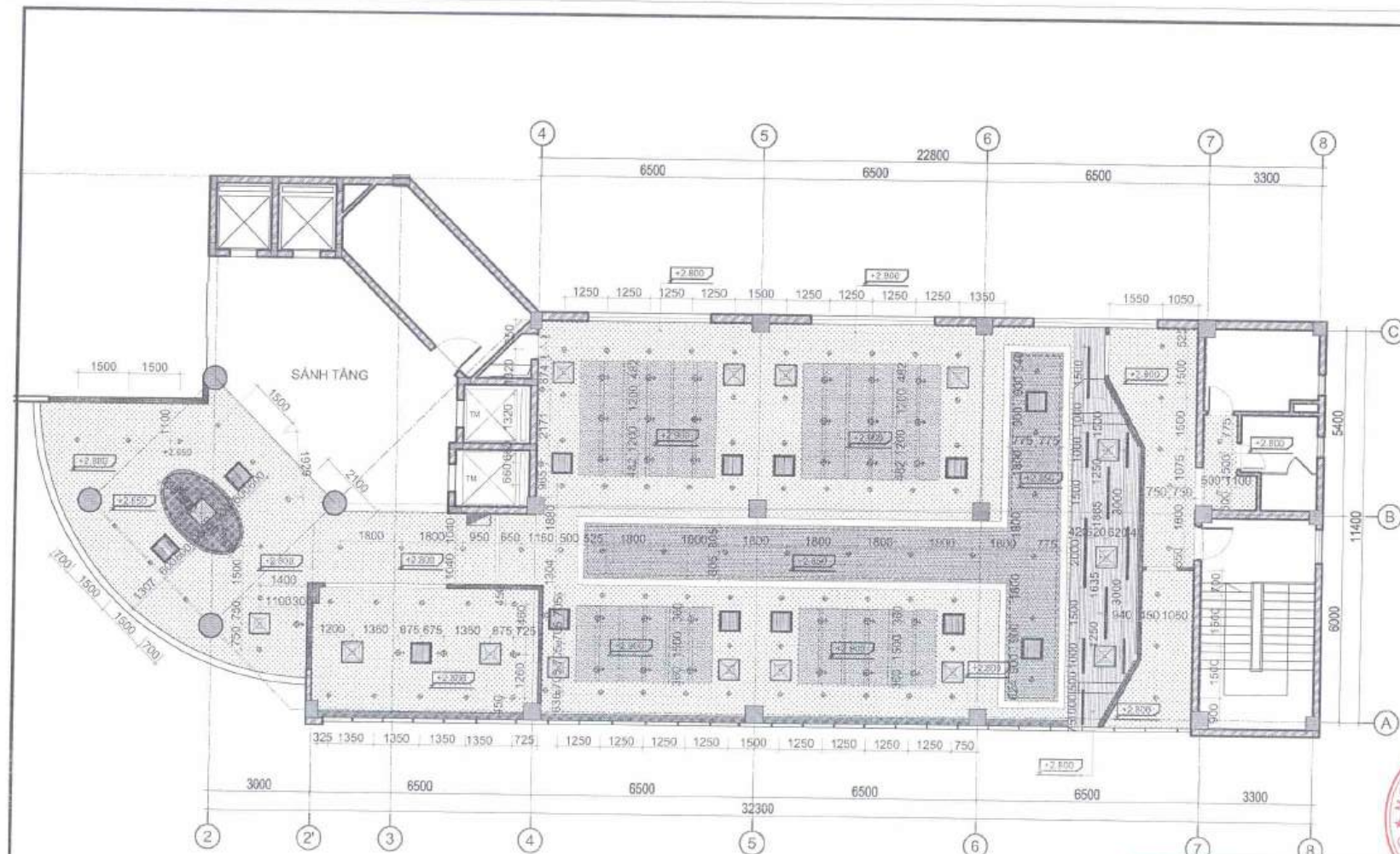
MẶT BẰNG ĐỊNH VỊ ĐỀN
