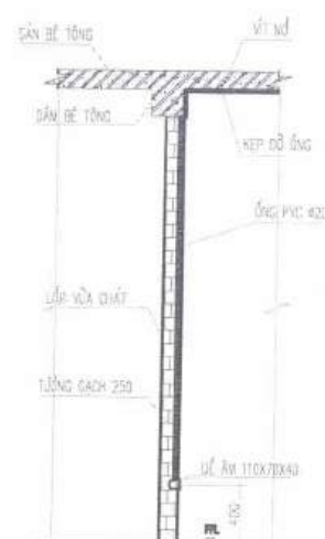
MẶT CẮT
