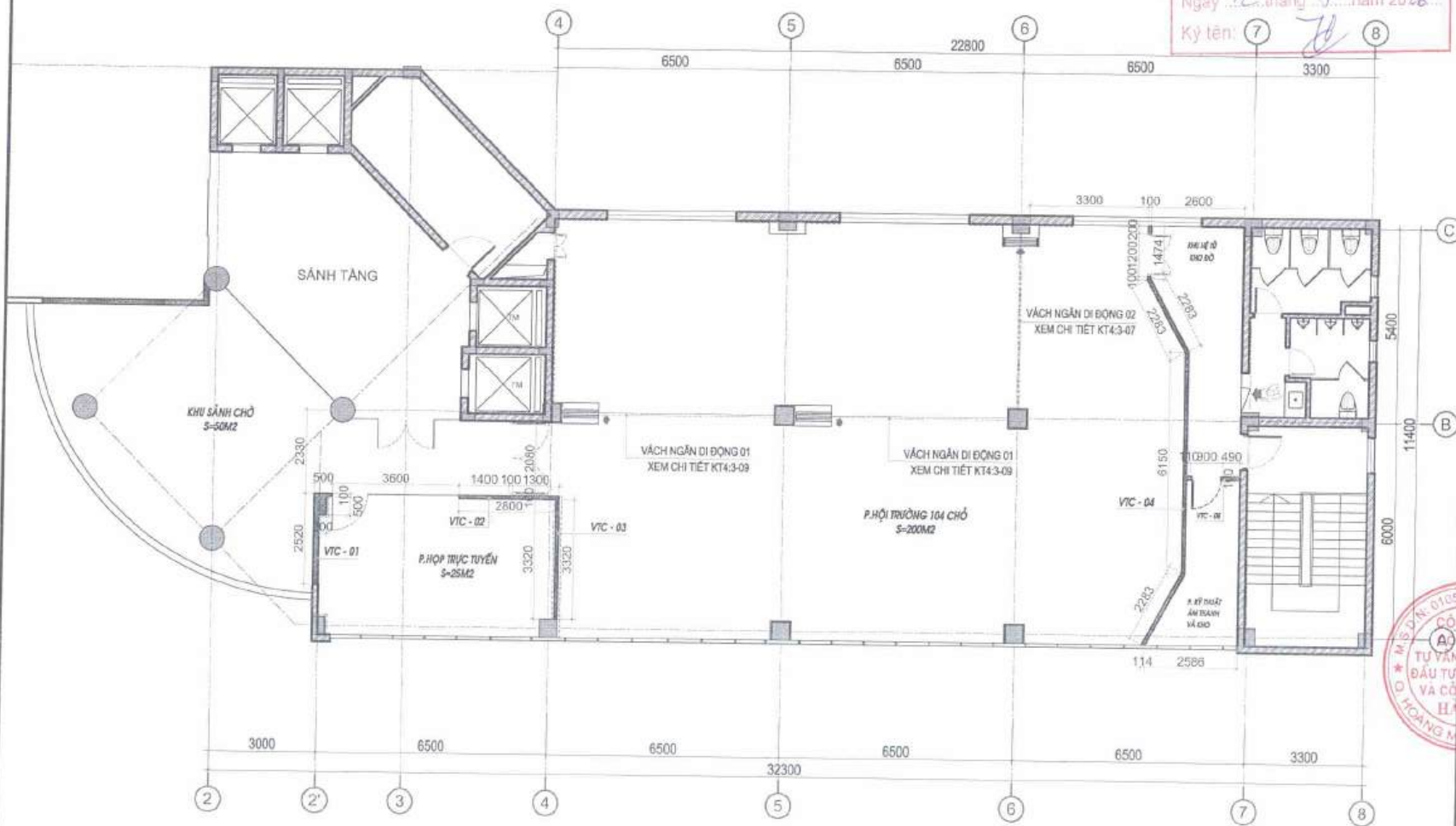
MẶT BẰNG ĐỊNH VỊ VÁCH THẠCH CAO BỔ SUNG TẦNG 4 DIỆN TÍCH XÂY DỰNG: 320M2
