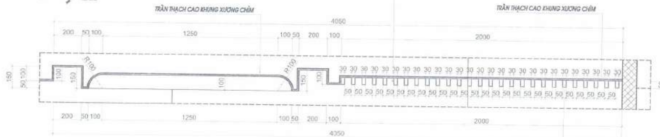
CHI TIẾT TRẦN THẠCH CAO 02
