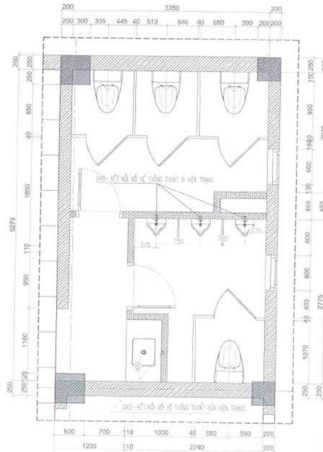
MẶT BẰNG THOÁT NƯỚC
