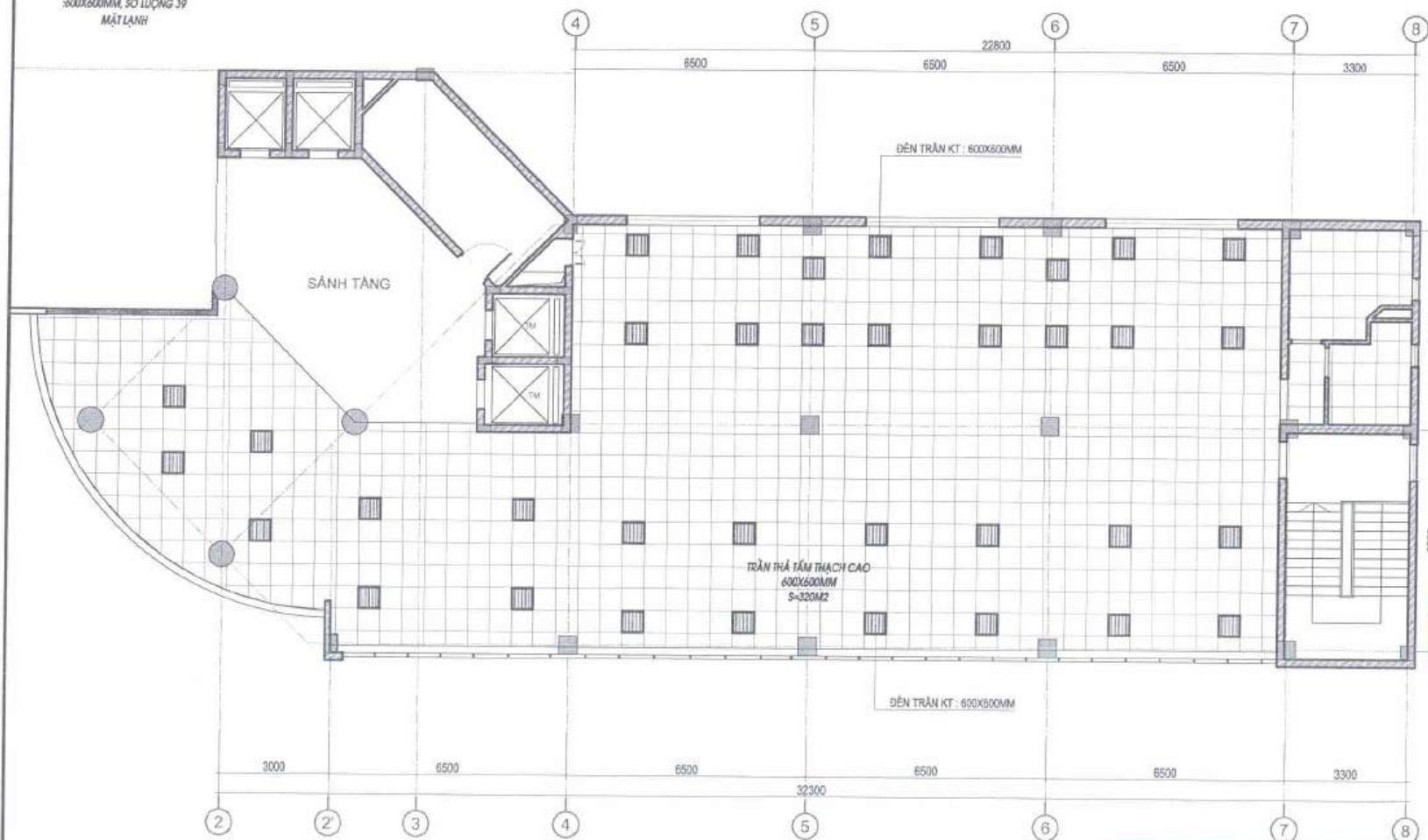
MẶT BẰNG ĐÈN TRẦN HIỆN TRẠNG TẦNG 4 DIỆN TÍCH XÂY DỰNG: 320M2
