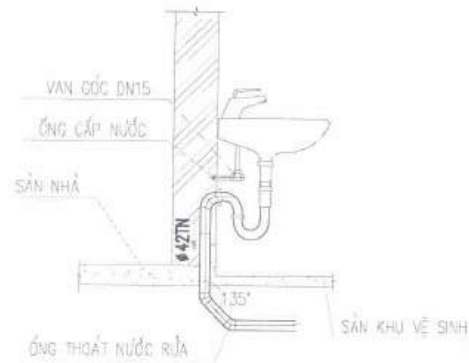
CHI TIẾT LẮP ĐẶT CHẬU RỬA
