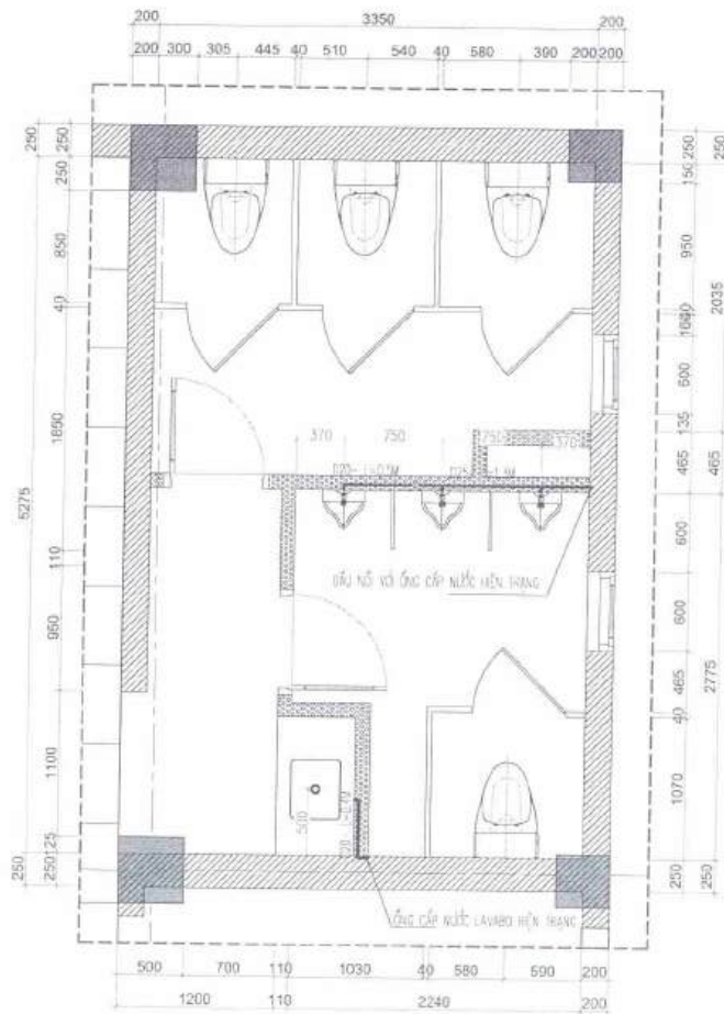
MẶT BẰNG CẤP NƯỚC
