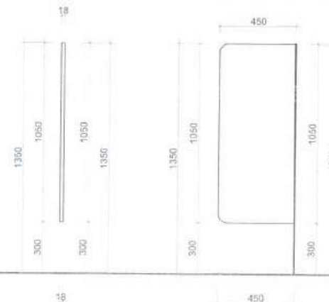
MẶT ĐỨNG
