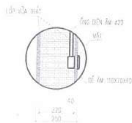
CHI TIẾT Ở CẮM TƯỜNG 250
