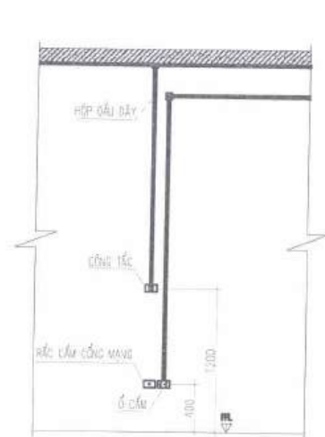
MẶT ĐÚNG
