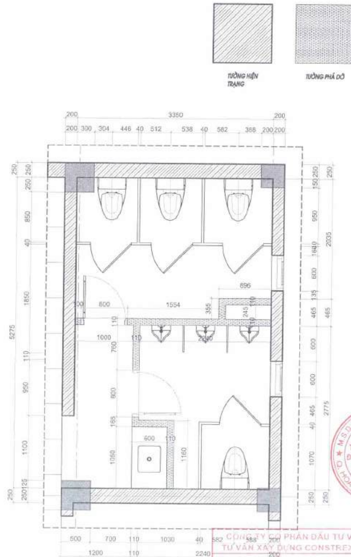
MẶT BẰNG XÂY MÓI
