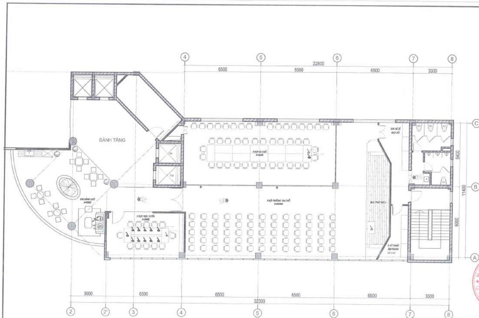
BỐ TRÍ MICRO HỘI HỢP TẦNG 4 DIỆN TÍCH XÂY DỰNG: 320M2
