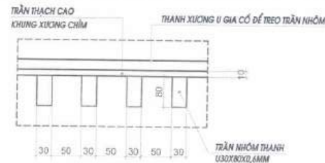
CHI TIẾT CẤU TẠO
