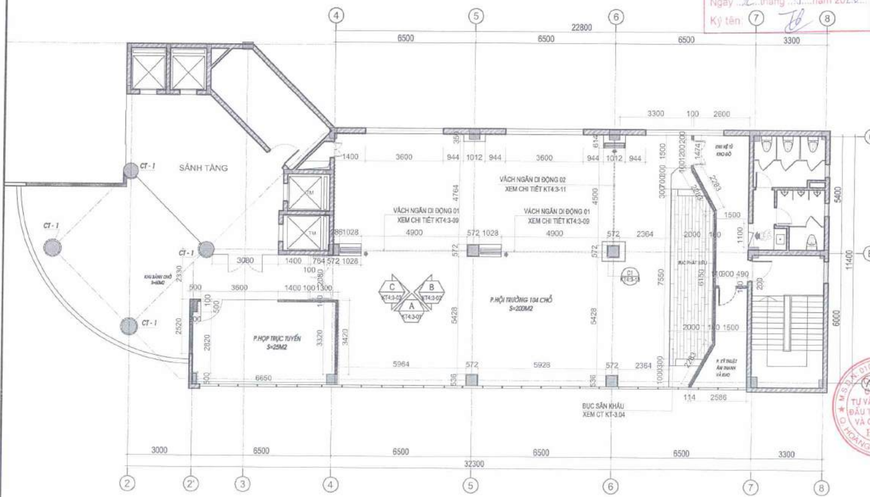
MẶT BẰNG KÍCH THƯỚC HOÀN THIỆN TẦNG 4 DIỆN TÍCH XÂY DỰNG: 320M 2
