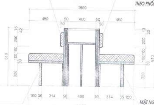
MẶT BÊN
