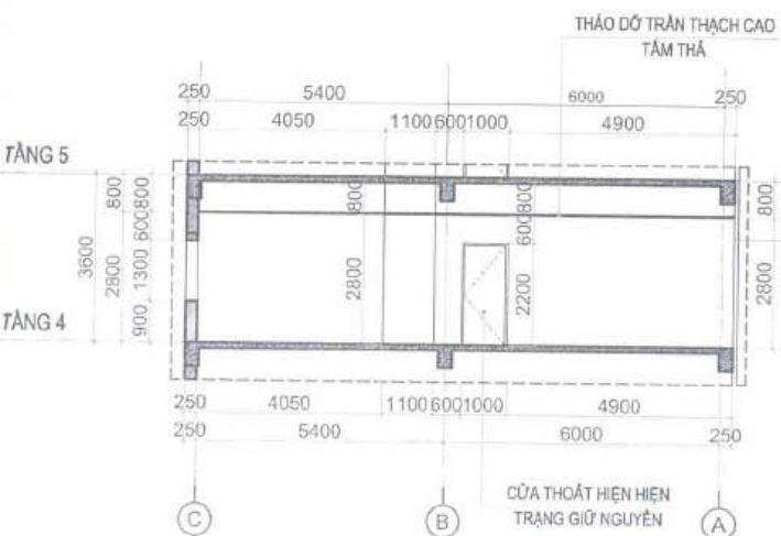
MẶT CẮT PHẪ ĐỒ 2-2
