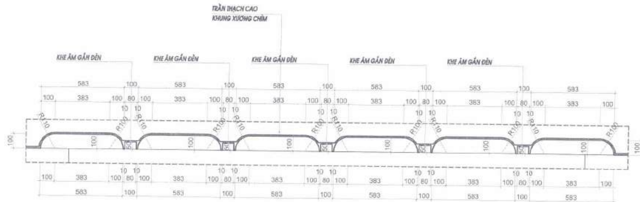
CHI TIẾT TRẦN THẠCH CAO 01
