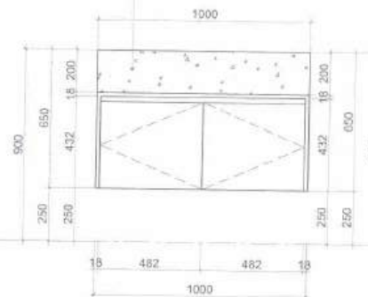
MẶT ĐÚNG
