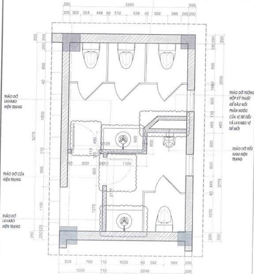
MẶT BẰNG PHÁ ĐỠ
