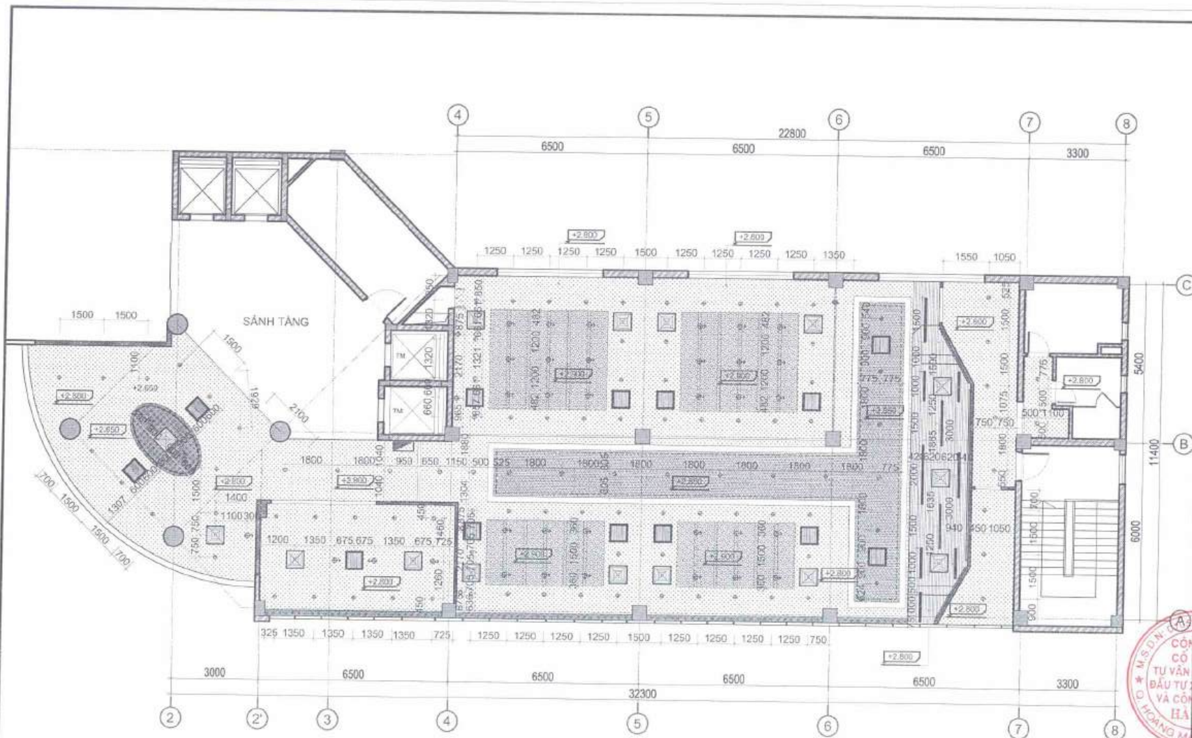
MẶT BẰNG ĐỀN TẦNG 4 DIỆN TÍCH XÂY DỰNG: 320M 2
