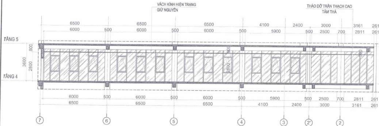
MẶT CẮT PHẪ DỠ 3-3
