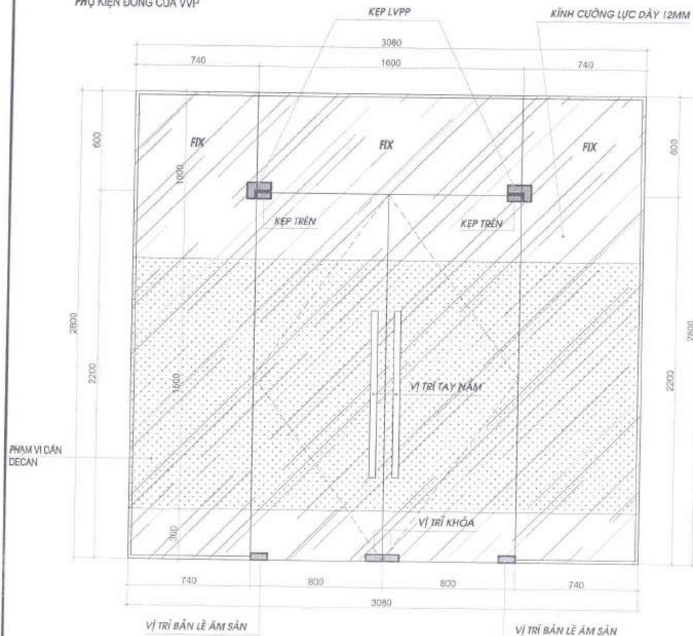
MẶT ĐÚNG CỬA
