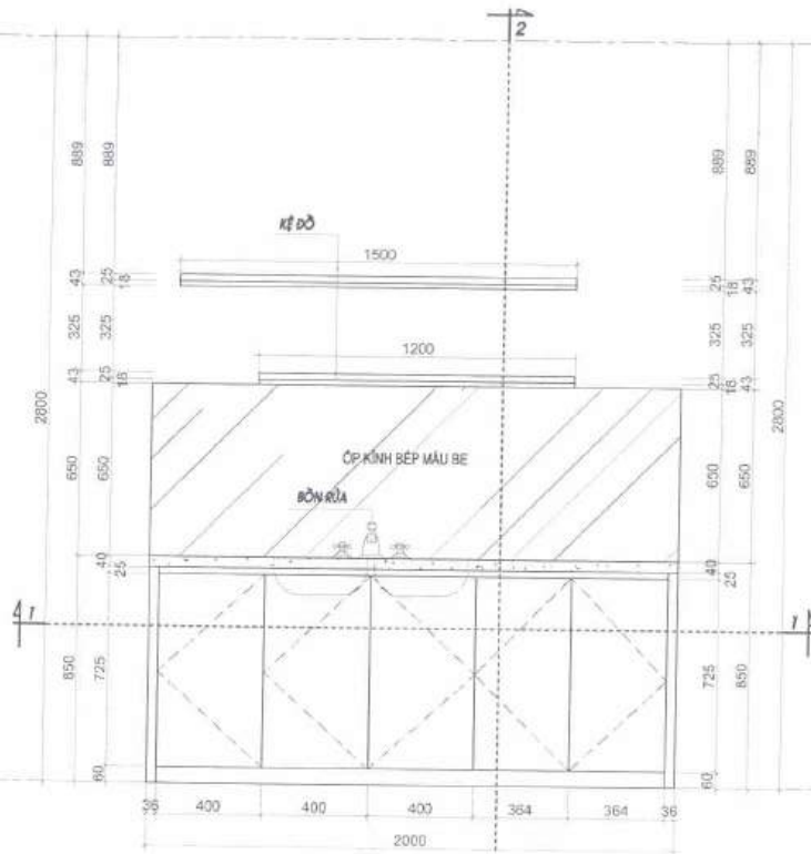
MẶT ĐÚNG
