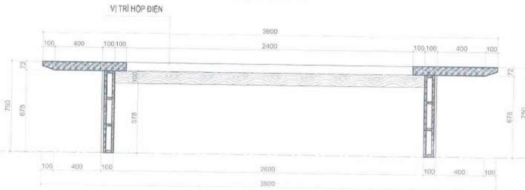
MẶT CẮT 1-1
