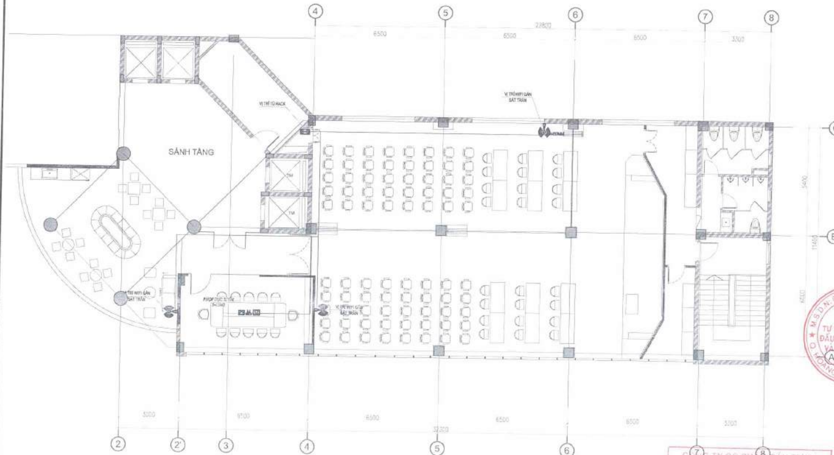
MẶT BẰNG ĐIỆN NHỆ TẦNG 4
