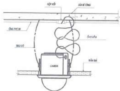
CHI TIẾT LẮP ĐẶT CAMERA DOME CỐ ĐỊNH ẨM TRẦN
