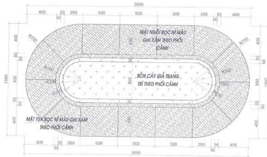
MẶT BẰNG
