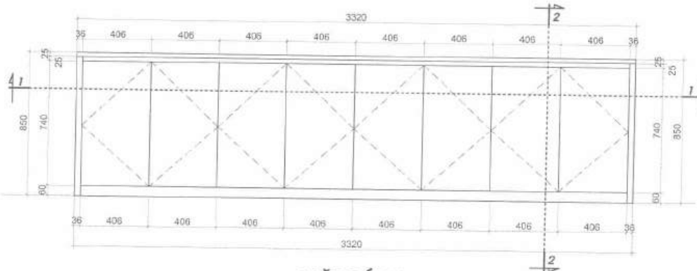
MẶT ĐÚNG
