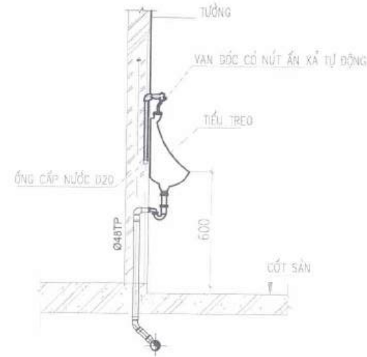
CHI TIẾT LẮP ĐẶT TIỂU NAM
