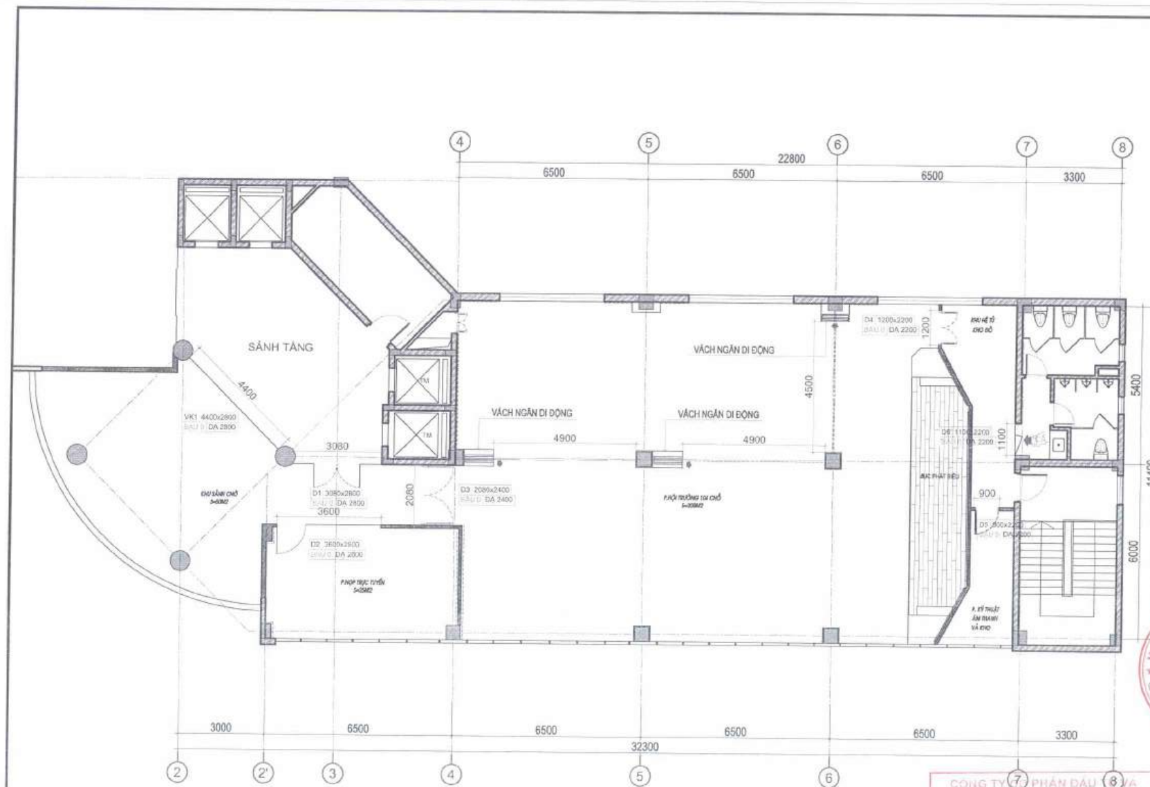
MẶT BẰNG ĐỊNH VỊ CỬA TẦNG 4 DIỆN TÍCH XÂY DỰNG: 320M 2
