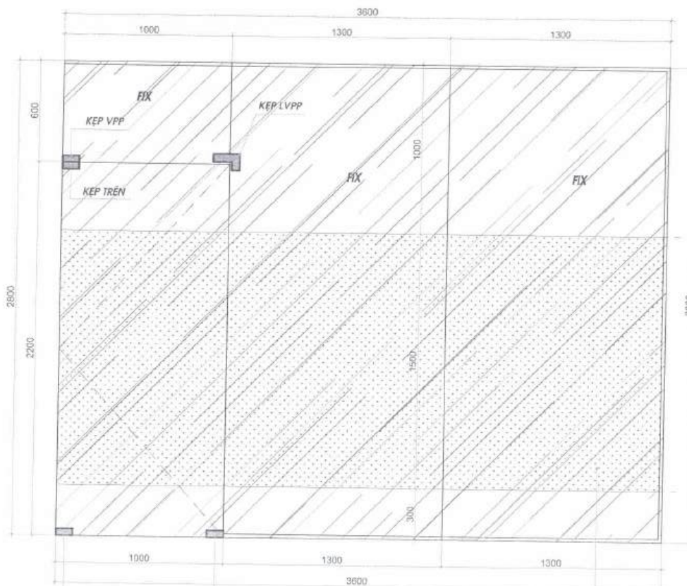
MẶT ĐÚNG CỬA
