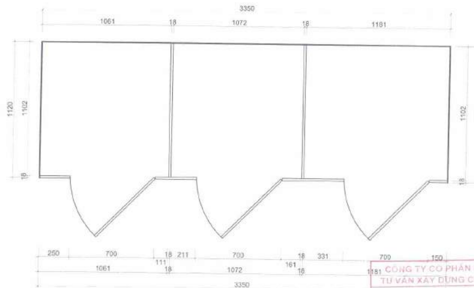
MẶT BẰNG
