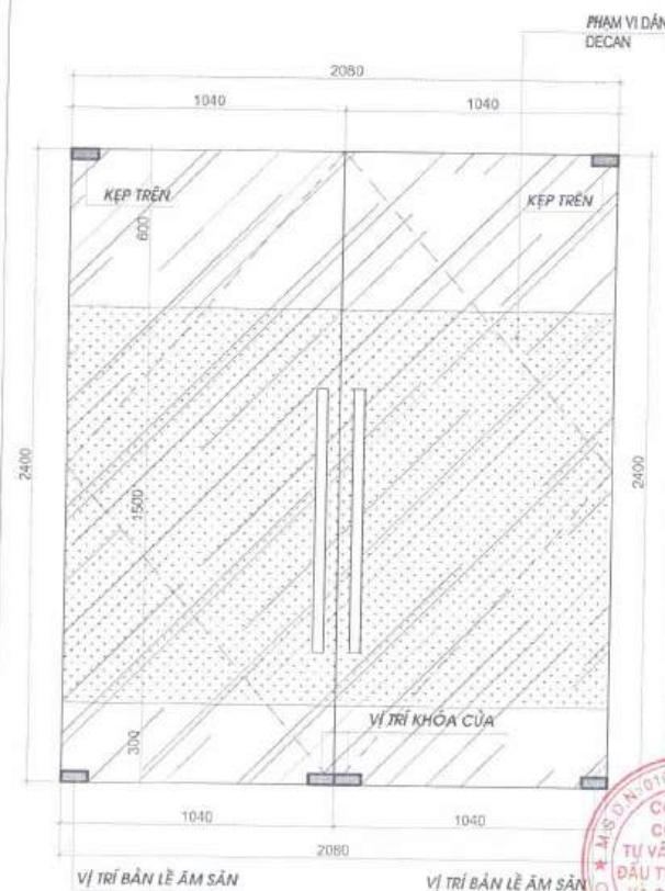
MẶT ĐÚNG CỬA
