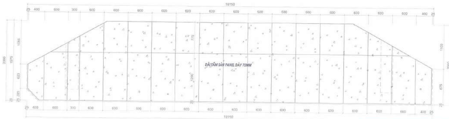
MẶT BẰNG TẤM SÀN PANEL KHU SÂN KHẤU
