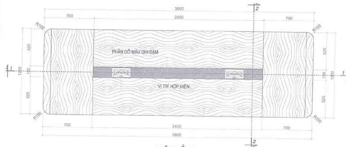
MẶT BẰNG
