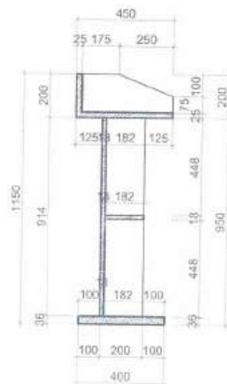
MẶT CẮT 2-2
