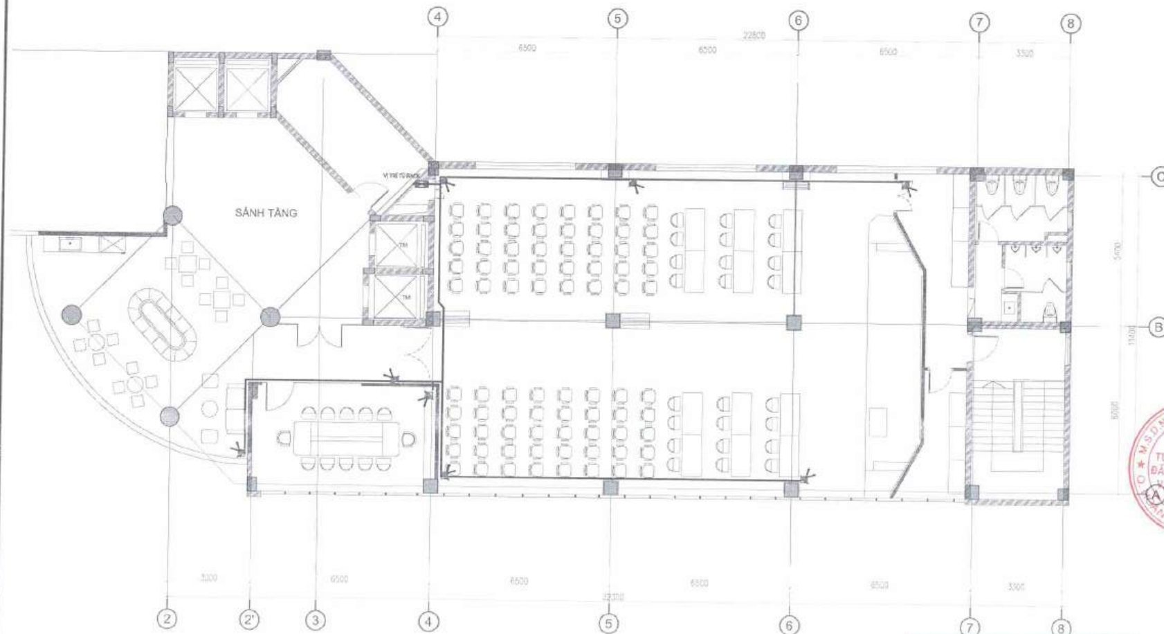
MẶT BẰNG ĐỊNH VỊ CAMERA TẦNG 4
