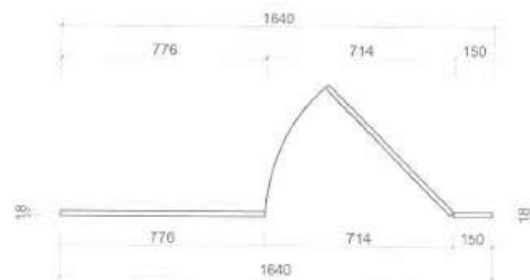
MẶT BẰNG
