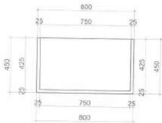
MẶT BẢNG
