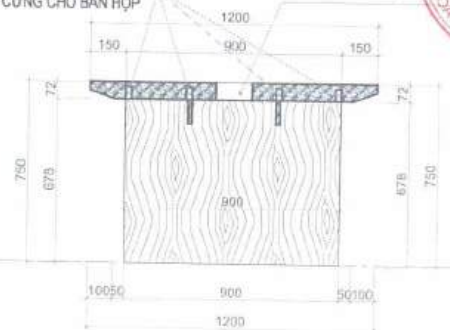
MẶT CẮT 2-2
