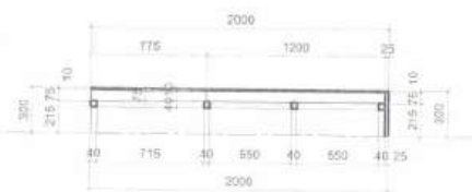
MẶT CẮT 2-2 KHU SÂN KHẤU
