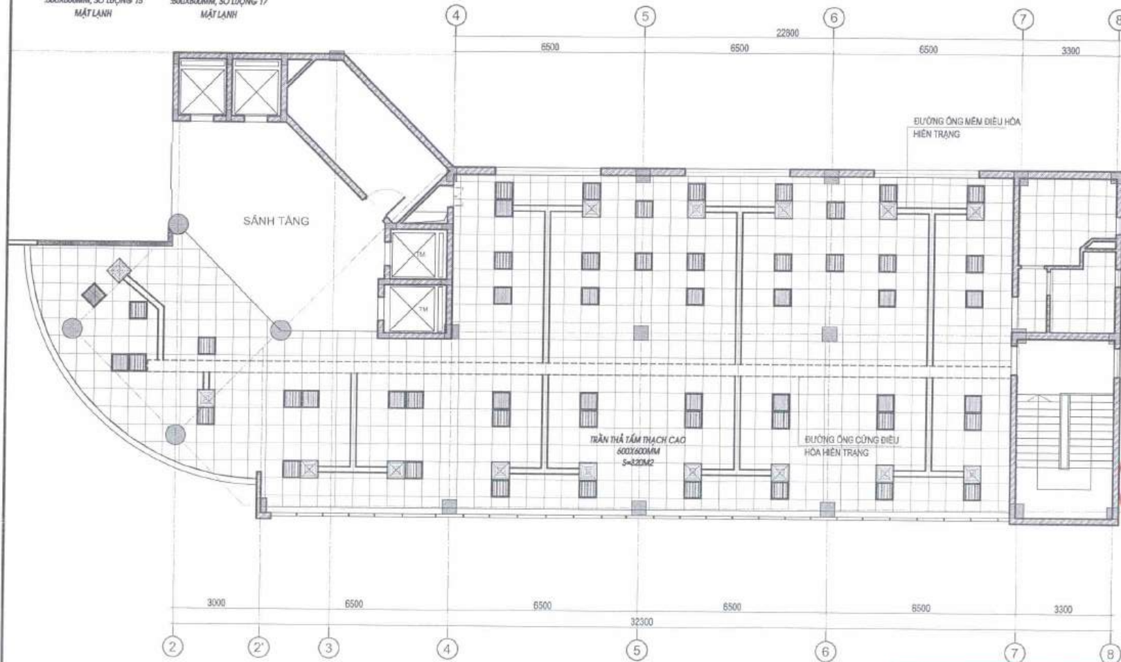
MẶT BẰNG TRẦN HIỆN TRẠNG TẦNG 4 DIỆN TÍCH XÂY DỰNG: 320M2
