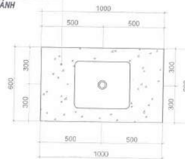
MẶT BẢNG
