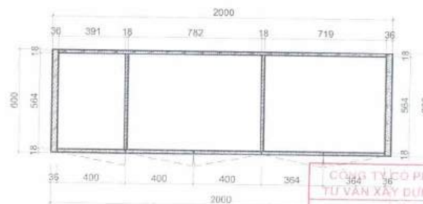
MẶT CẮT 1-1
