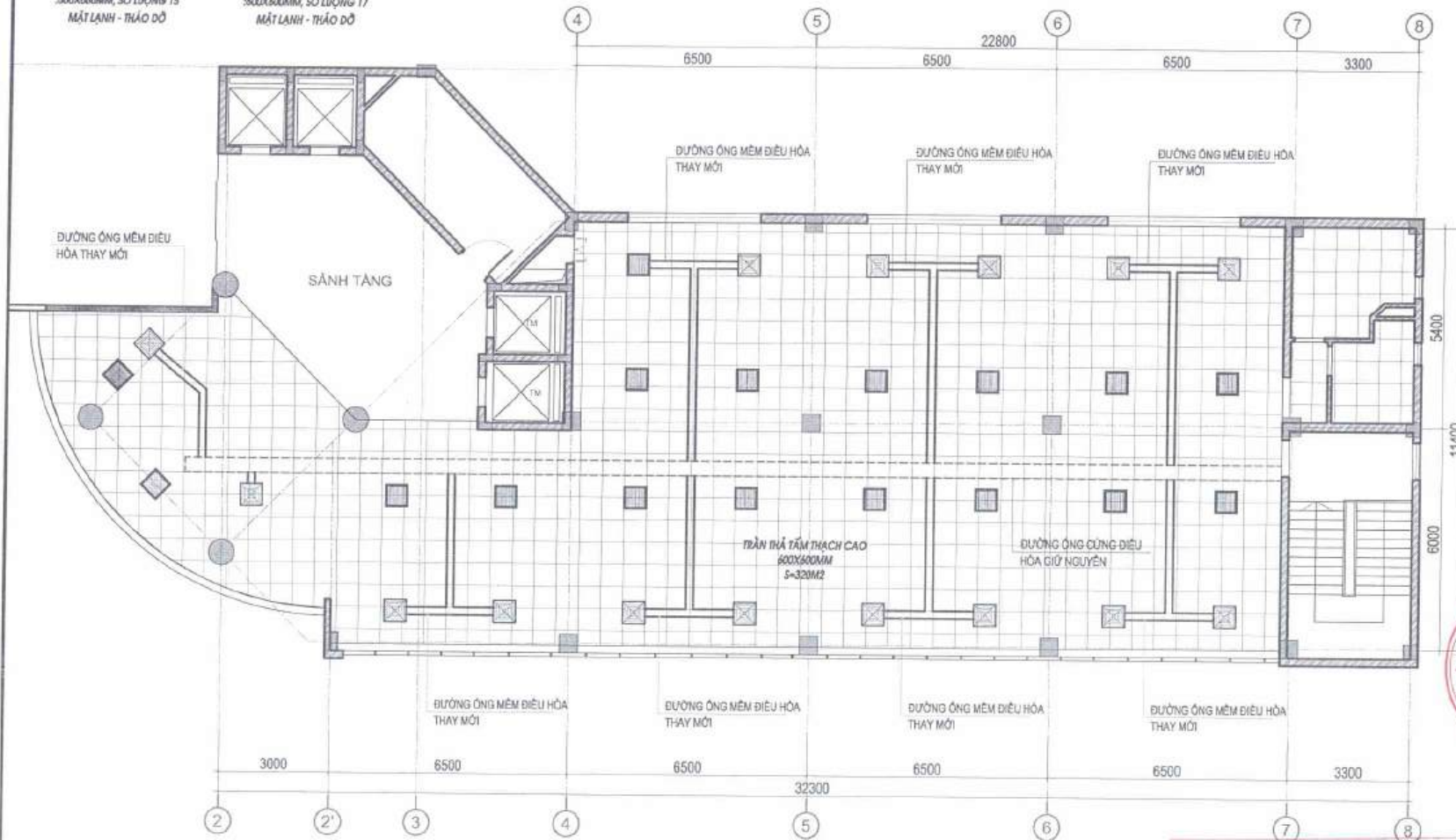
MẶT BẰNG THẢO DỒ TRẦN TẦNG 4 DIỆN TÍCH XÂY DỰNG: 320M2
