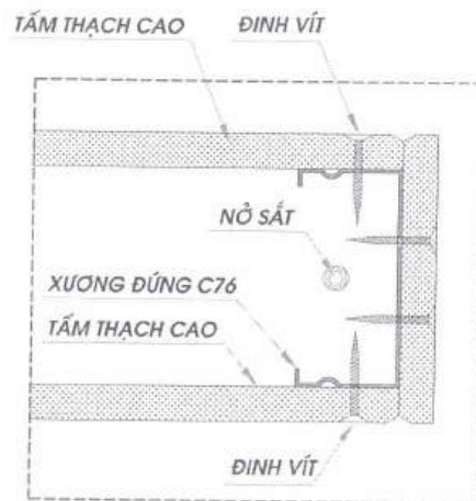
CHI TIẾT ĐẦU VÁCH
