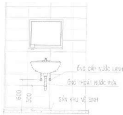
CHI TIẾT LẮP ĐẶT CHẬU RỬA
