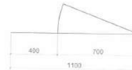
MẶT BẰNG CỬA
