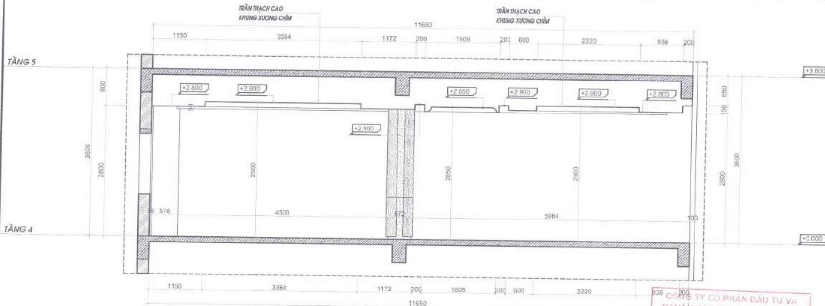
MẶT CẮT 3-3
