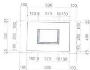
MẶT CẮT 1-1
