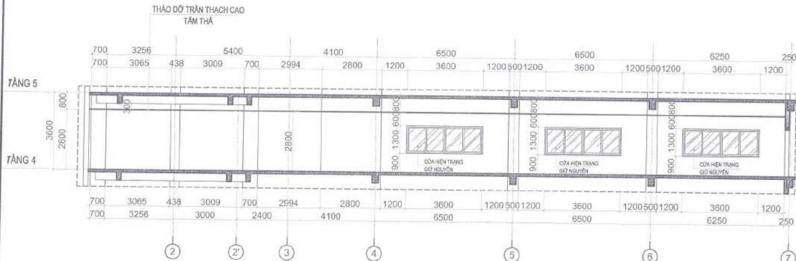
MẶT CẮT PHẪ ĐỒ 1-1
