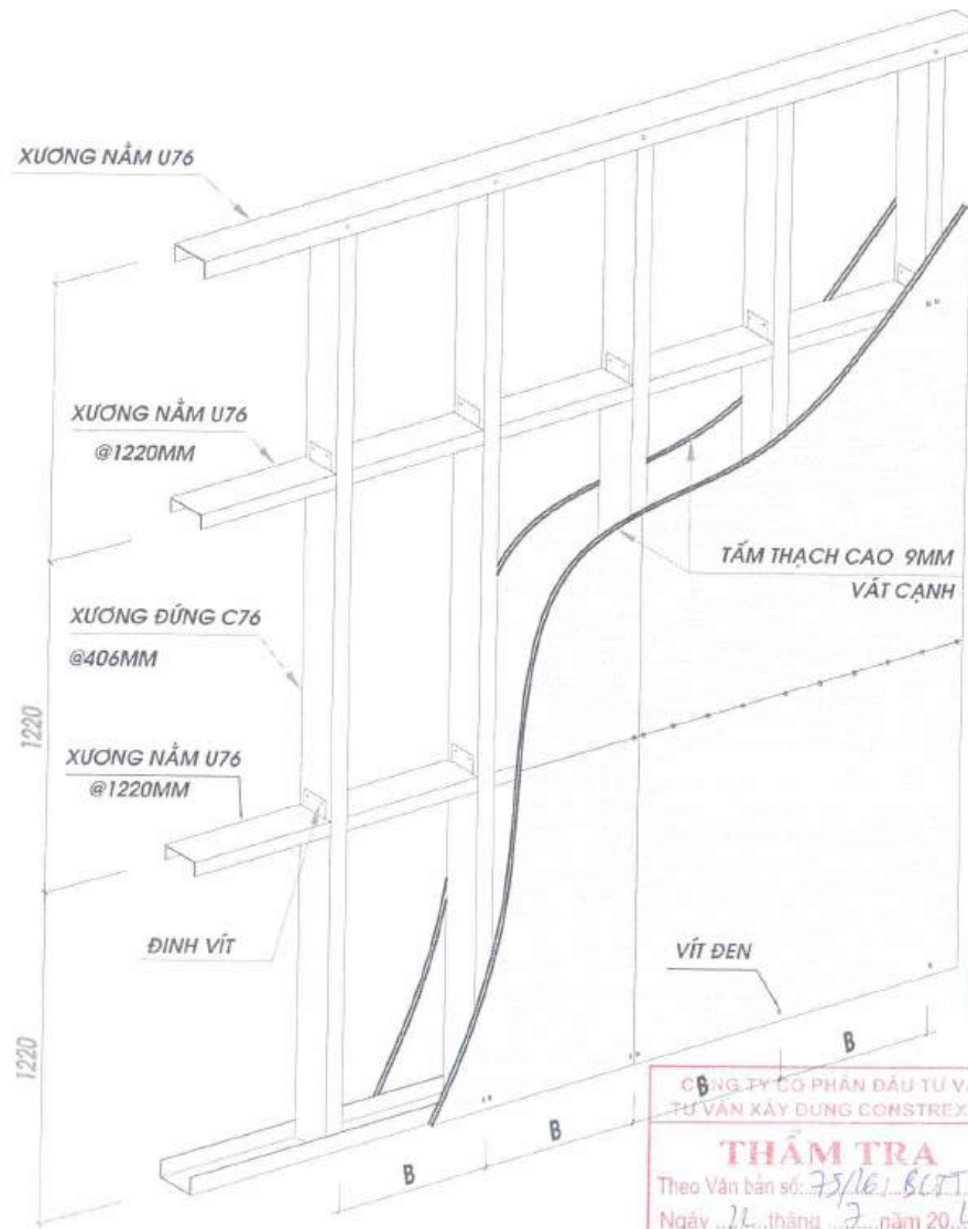
HỆ KHUNG VÁCH THẠCH CAO ĐIỂN HÌNH
