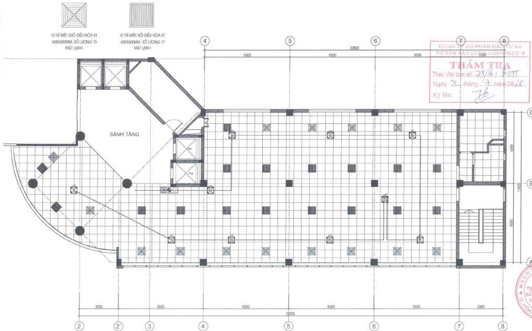
MẶT BẰNG BẢO CHÁY HIỆN TRẠNG TẦNG 4 DIỆN TÍCH XÂY DỰNG: 320M2
