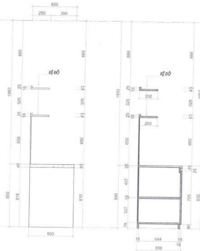
MẶT BÊN
