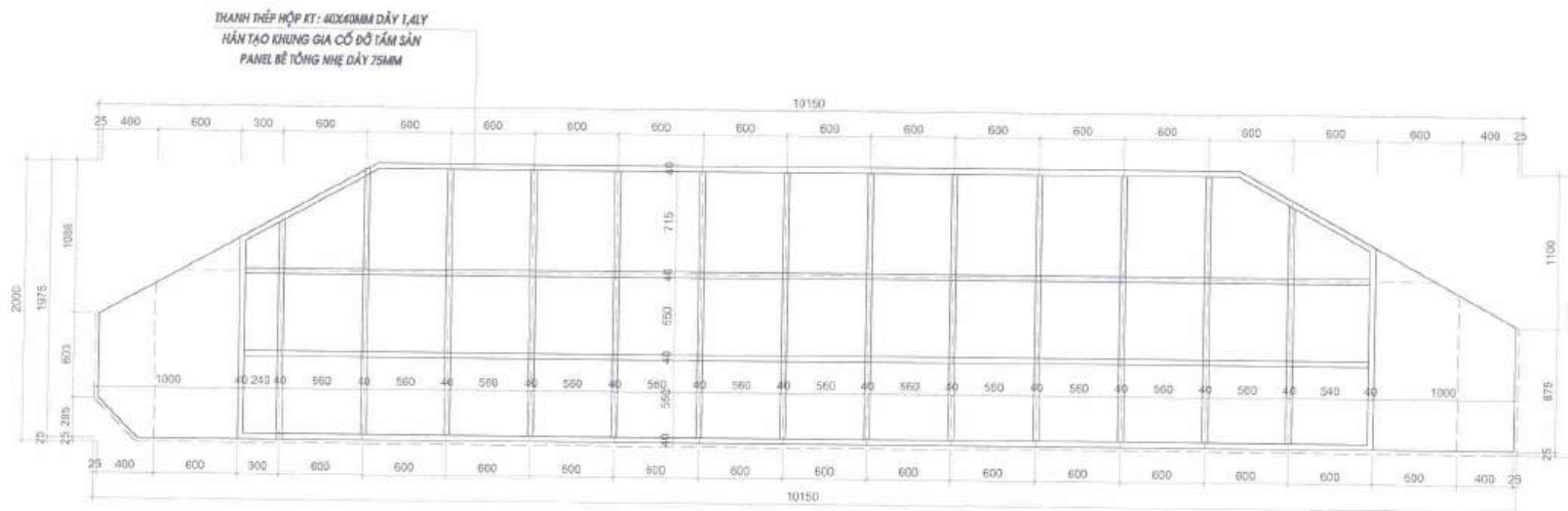
MẶT BẰNG KHUNG TẤM PANEL KHU SÂN KHẤU
