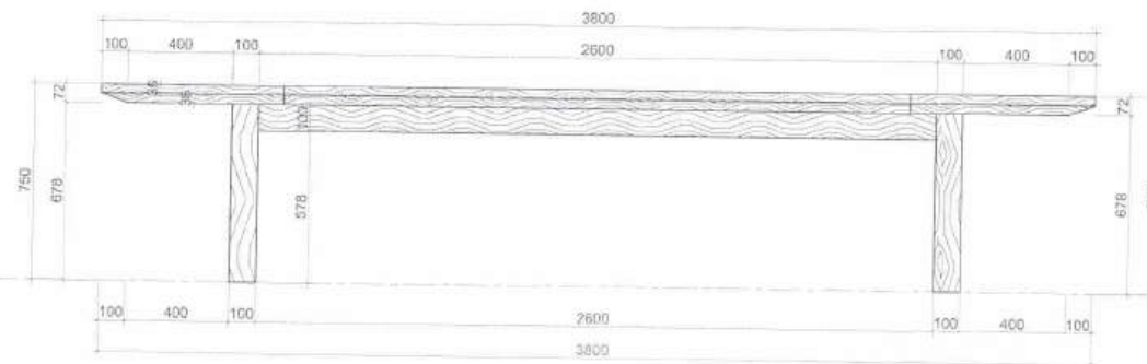
MẶT ĐÚNG
