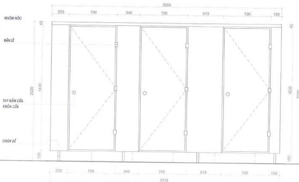
MẶT ĐỨNG
