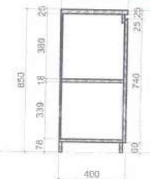
MẶT CẮT 2-2
