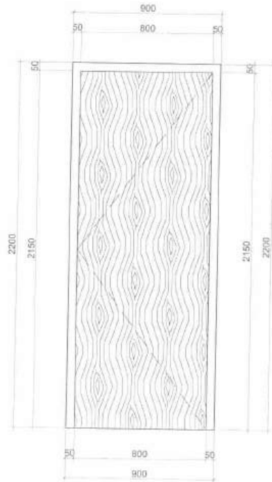
MẶT ĐÚNG CỬA
