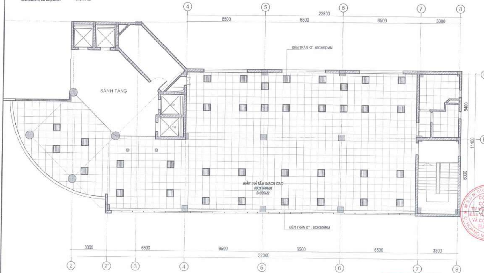
MẶT BẰNG THẢO DỜ ĐÈN TRẦN TẦNG 4 DIỆN TÍCH XÂY DỰNG: 320M 2
