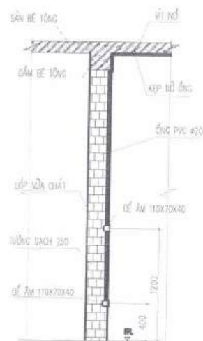
MẶT CẮT
